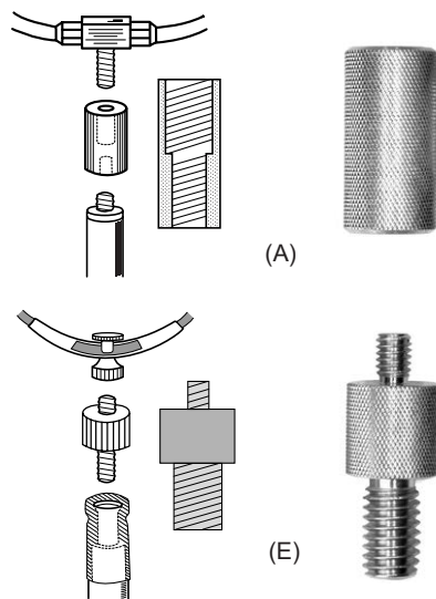
ジョイント金具
